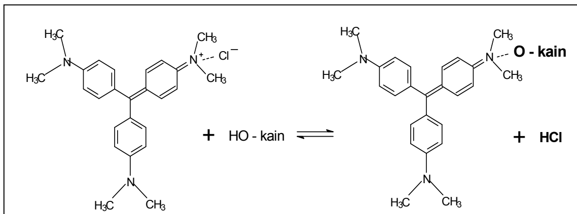
Gambar 2. Reaksi MV dan Serat Kain secara Elektrostatis Melepaskan Proton
