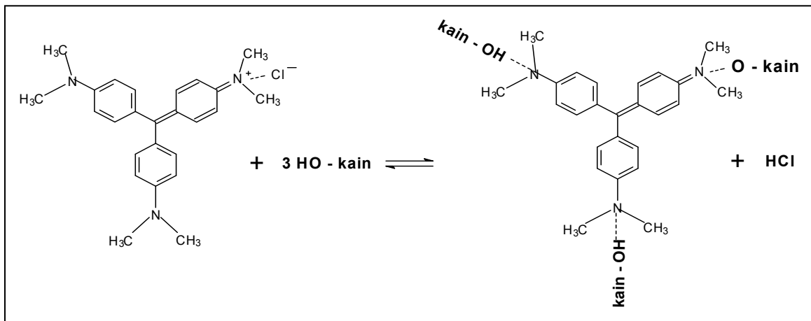
Gambar 4. Pola Ikatan MV dan Serat Kain yang Multibonding , Mengikuti Persamaan Freundlich
