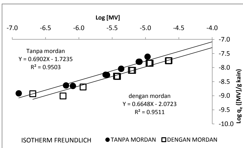
Gambar 3. Pola Ikatan MV dan Serat Kain Mengikuti Persamaan Freundlich
