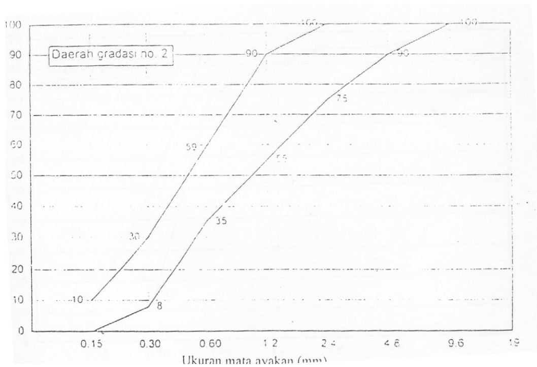
Grafik 4 Batas Gradasi Pasir (Sedang) No. 2
