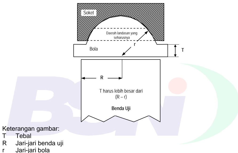
Gambar 1 - Sketsa landasan tekan yang dapat berputar
