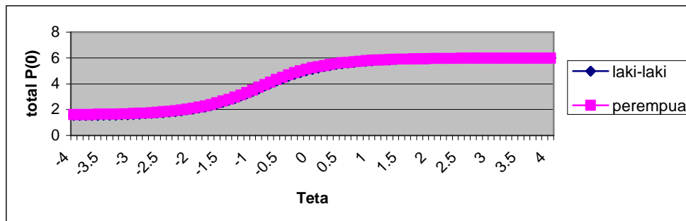
Gambar 1. Grafik Nilai Peluang Seluruh Butir Tes
