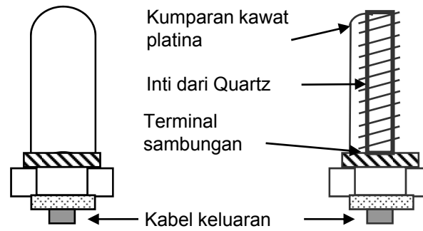
Gambar 2.9. Konstruksi RTD
