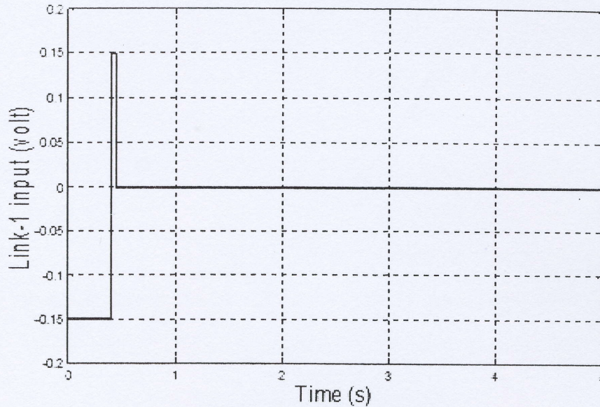
Gambar 2. Input Bang-bang
