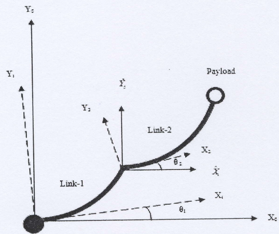
Gambar 1. Skema RLDL
