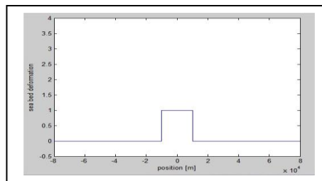
Gambar 3. Deformasi Persegi
