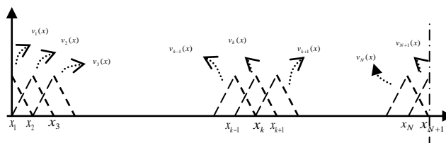
Gambar 1. Fungsi Tent
